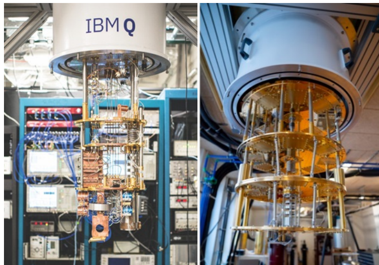
Рис. 3. Квантові комп'ютери а) IBM б) Intel
