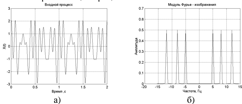
Рис. 1. Спектральный анализ.
