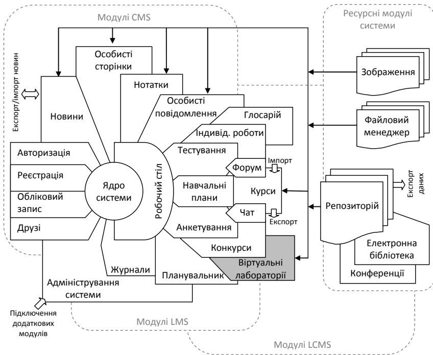
Рис. 2.9. Загальна структура системи «Агапа»
