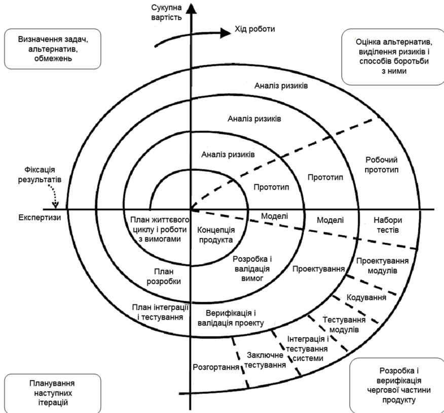
Рис. 2.6. Спіральна модель процесу розробки програмного забезпечення (за Б. Боемом [26])
