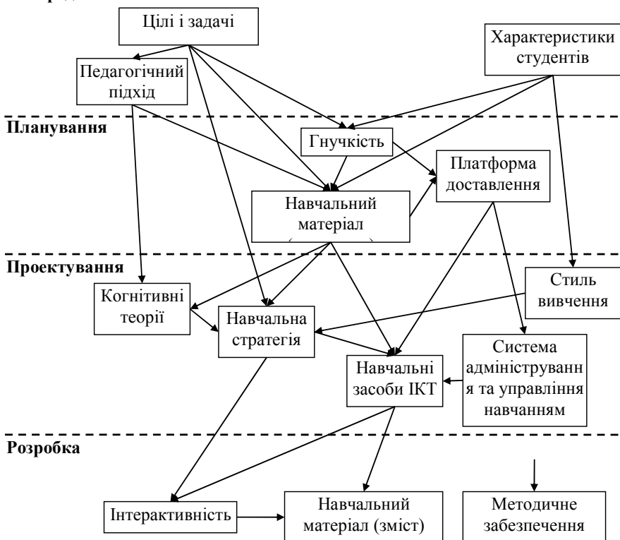
Рис. 2.2. Схема взаємного впливу компонентів системи навчання і послідовності прийняття проектних рішень (за В. І. Гриценком [127])
