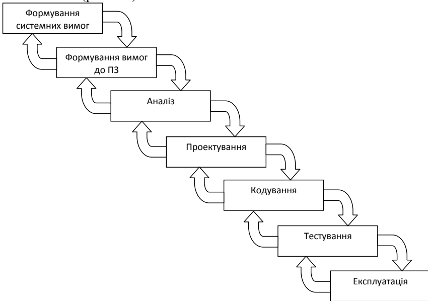
Рис. 2.5. Ітеративна модель розробки програмного забезпечення (за [81])
