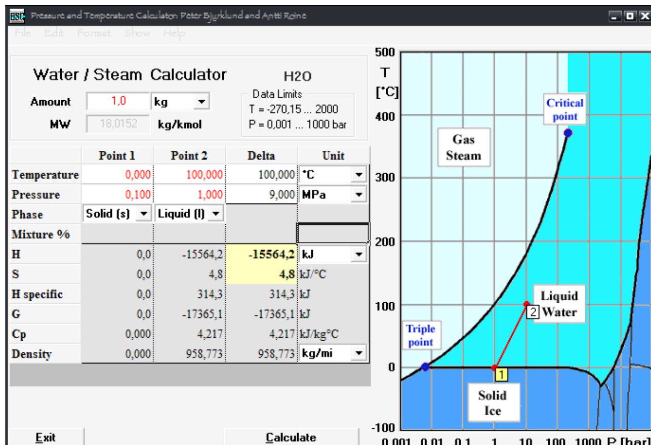
Рис. 2.32. Вікно програми HSC Chemistry 5.1, у якому на фазовій діаграмі води моделюються її агрегатний стан і термодинамічні характеристики у залежності від температури і тиску
