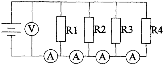
Рис.6 Паралельне підключення споживачів
