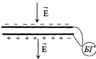
Рис. 1. Повітряний конденсатор
