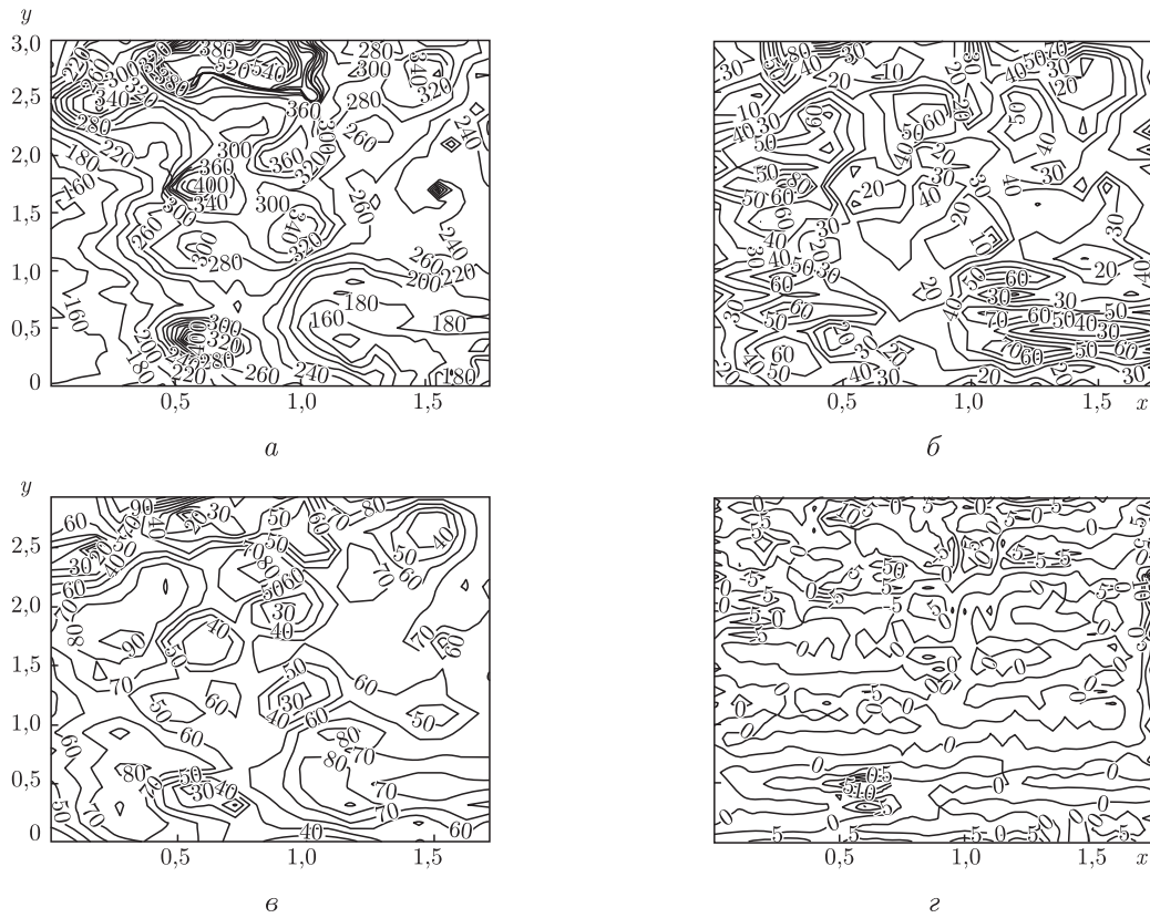
Рис. 2. Результаты решения обратной нелинейной задачи магнитометрии: а : Карта неосредненного магнитного поля Z_a участка 1 (обозначения те же). б : Карта глубин H_1 до верхней поверхности первого слоя (изолинии, м). в : Карта глубин H_2 до верхней поверхности второго слоя. г : Карта остатков магнитного поля (сечение изолиний 5 нТл)
