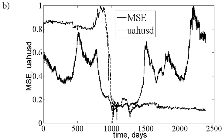
Рис. 1. Порівняльна динаміка валютних курсів з відповідною мультимасштабною ентропією для (а) eurUSD – євро - дол. США, (б) uahUSD – українська гривня – дол. США
