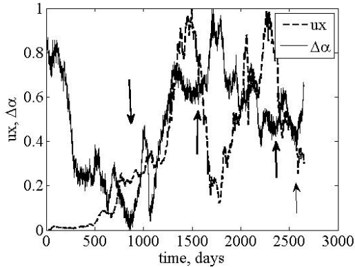
Рис. Зміна з часом ентропії перестановок (а) та ширини спектру сингулярності (b) для індексу іх у різні за волатильністю періоди часу. Розрахунки проведені для ширини вікна у 1000 точок з кроком в один день. Стрілками відмічені періоди відомих кризових явищ
